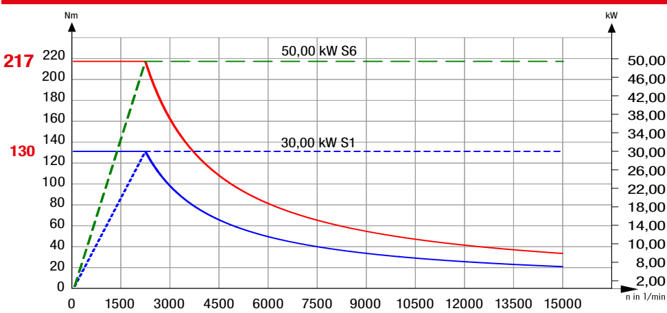
HSK A63, CELOX 15000 1/min, 217 Nm, 50,00 kW
