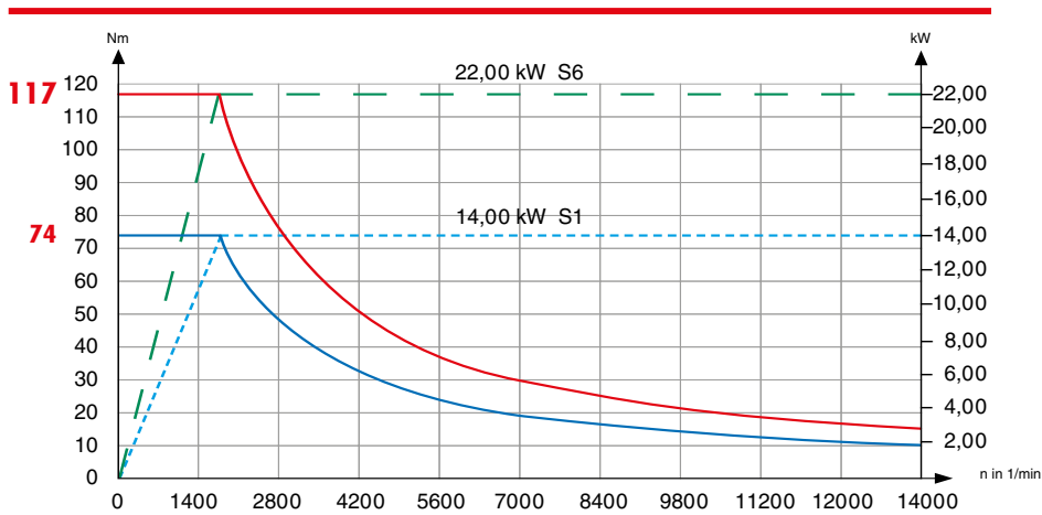
CELOX 14000 1/min 29,00 kW*
