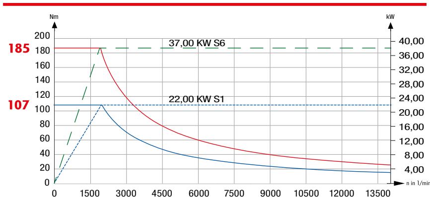
CELOX 14000 1/min 37,00 kW*
