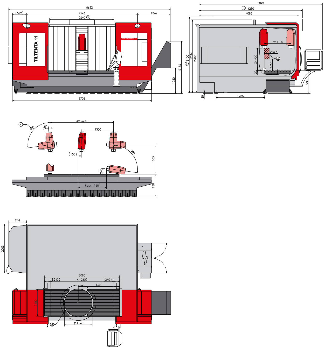
Zeichnungen unverbindlich. Maße können sich ändern und dienen als Richtwert. [Illustrations are not binding. Dimensions are subject to change and serve for orientation purpose.] Abbildung zeigt die TILTENTA 11 mit dem Magnum-Werkzeugmagazin für 65 Werkzeuge und mit einem Kratzbandspäneförderer. [Figure shows the TILTENTA 11 with magnum tool magazine for 65 tools and with scraper belt chip conveyor.]
