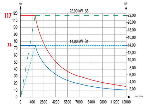
12000 1/min 22,00 kW
