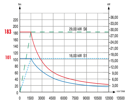
12000 1/min 29,00 kW
