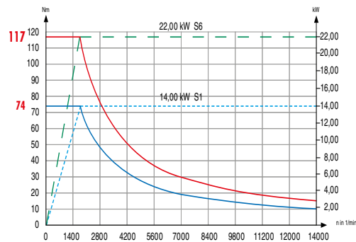
14000 1/min 22,00 kW
