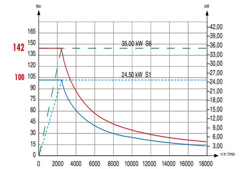
18000 1/min 35,00 kW
