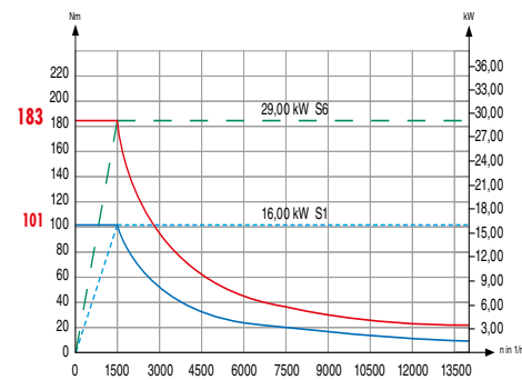
14000 1/min 29,00 kW
